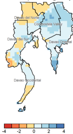
SPEI3 (Jul-Aug-Sep)
